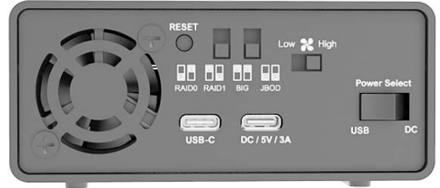
後面部
